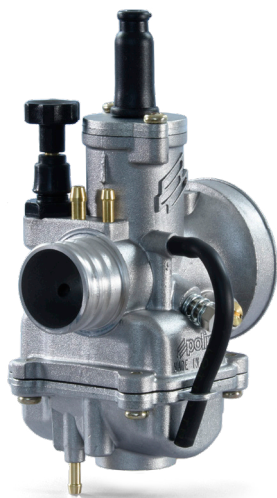
201.1500 UNIVERSAL
