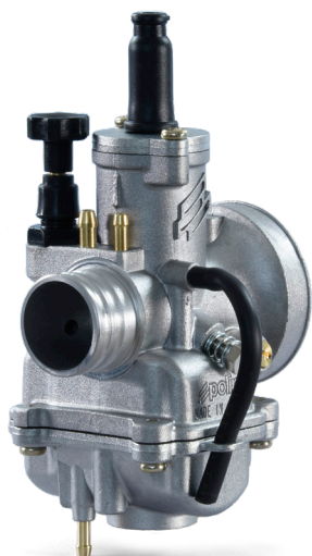
201.2300 UNIVERSAL
