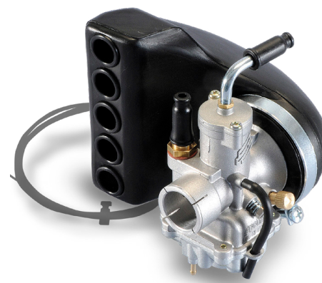
201.1905 VESPA
