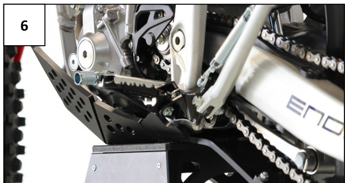
6 Fix the N°36 plate with : / Fixer la plaque N°36 avec: 2 Tfhc 6x25mm + 2 M6 Washers + 2 Em6f
