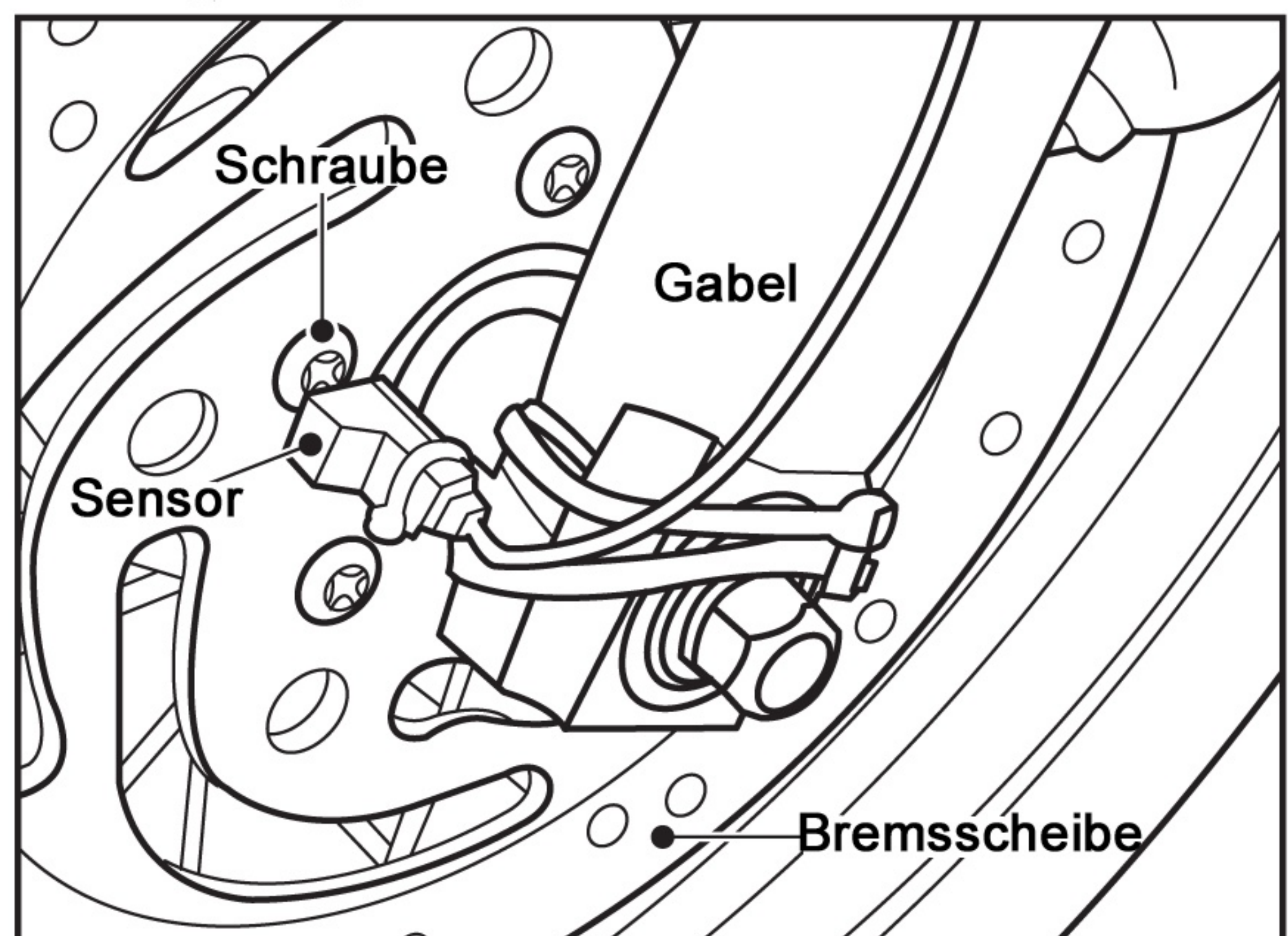
Montagebeispiel
