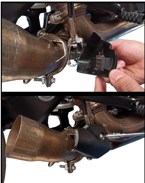
FISSAGGIO COVER ORIGINALE ORIGINAL COVER MOUNTING
