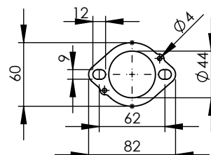
S.s Flange 112A cod.204569 Sp.5mm
