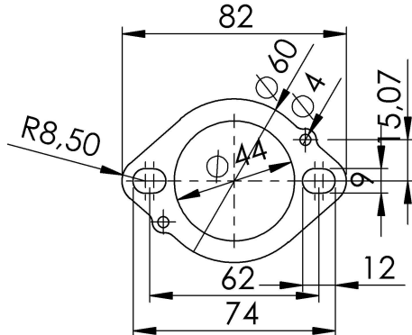
S.s. Flange Cod.204448R
